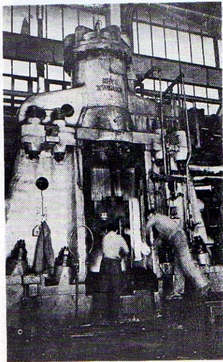
Kováči pri zápusťkovom kovaní.
